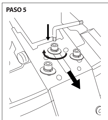
PASO 5 Tirar del respaldo hacia atrás hasta que los tornillos hagan tope con el mecanismo y ajustar
