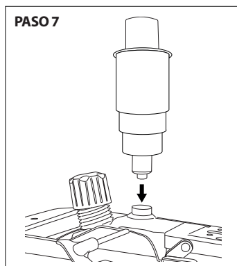
PASO 7 Colocar la columna neumática en el orificio de la base del mecanismo.
