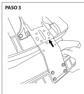
PASO 3 Insertar el soporte del respaldo en el mecanismo
