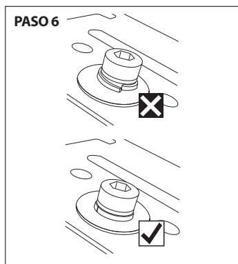
PASO 6 Ajustar los tornillos hasta que las arandelas Grower queden planas.
