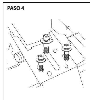
PASO 4 colocar los 3 tornillos que habían sido retirados y atornillarlos sin ajustar.
