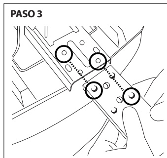
PASO 3 Insertar el soporte del respaldo en el mecanismo hasta que los 4 posicionadores queden alineados
