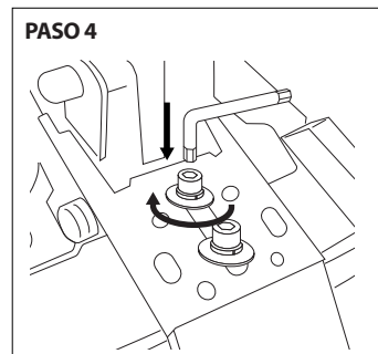
PASO 4 Colocar los 2 tornillos que habían sido retirados del respaldo y ajustar
