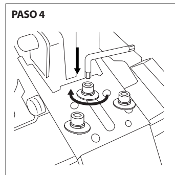
PASO 4 Colocar los 3 tornillos que habían sido retirados del respaldo y ajustar
