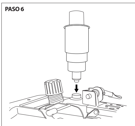
PASO 6 Colocar la columna neumática en el orificio de la base del mecanismo
