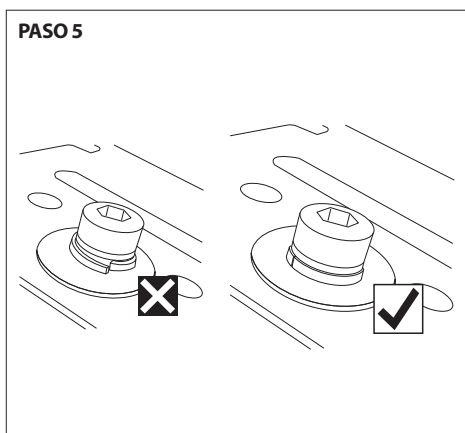
PASO 5 Ajustar los tornillos hasta que las arandelas Grower queden planas
